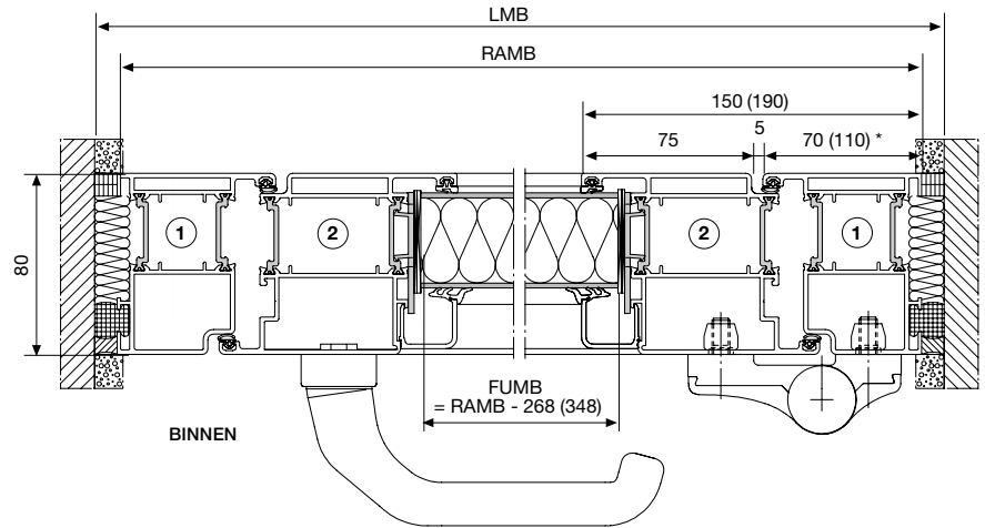
Horizontale doorsnede
